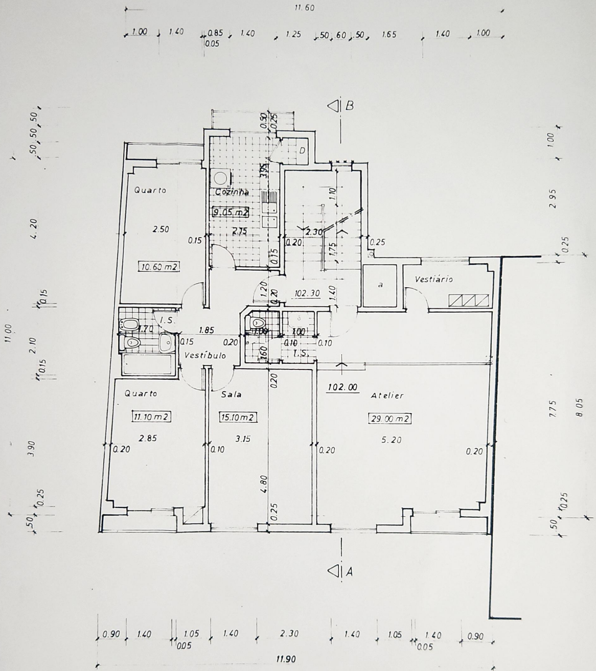
1º Andar
